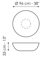
Planet Width: 96cm Depth: 96cm Height: 33cm
